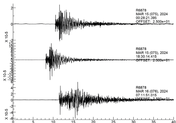
Sismogrames de terratrèmols amb epicentre prop de Vidreres del 15 de març a la 1:28 h (magnitud 2,3) i a les 19:30 h (magnitud 2,8), juntament amb el registre del terratrèmol (magnitud 3.0) del dia 16 amb epicentre al Baix Empordà.
